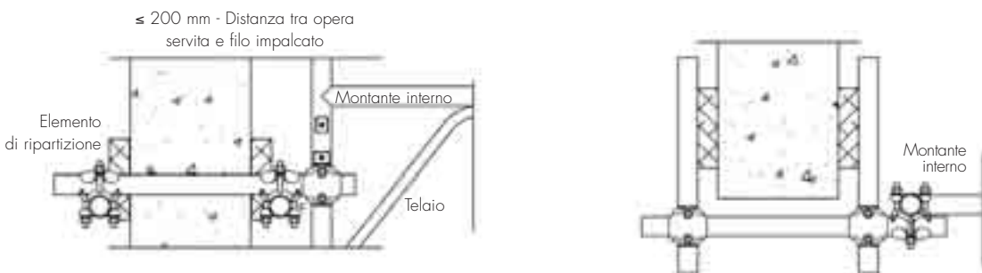
Fig. 9 - Esemio di ancoraggio "a cravatta"
